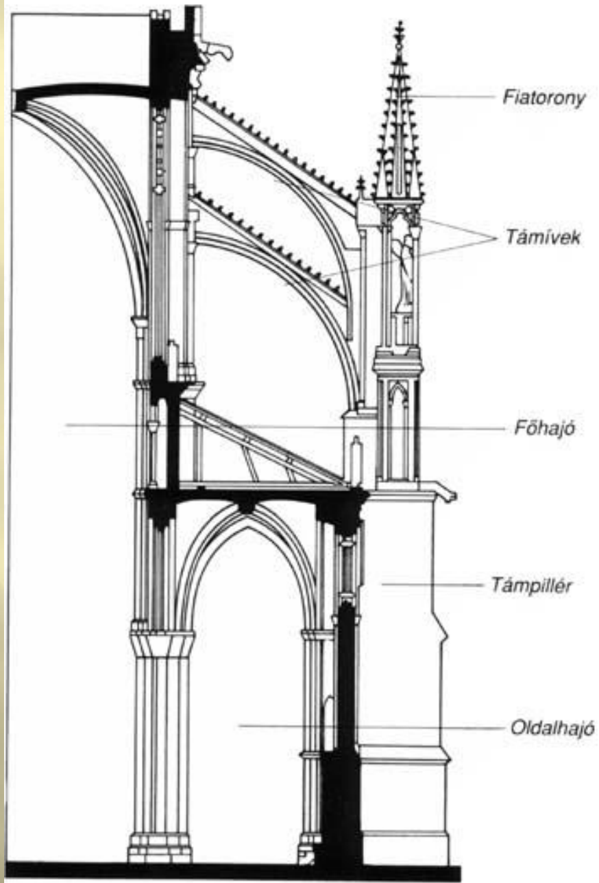
támív-támpillér rendszer
